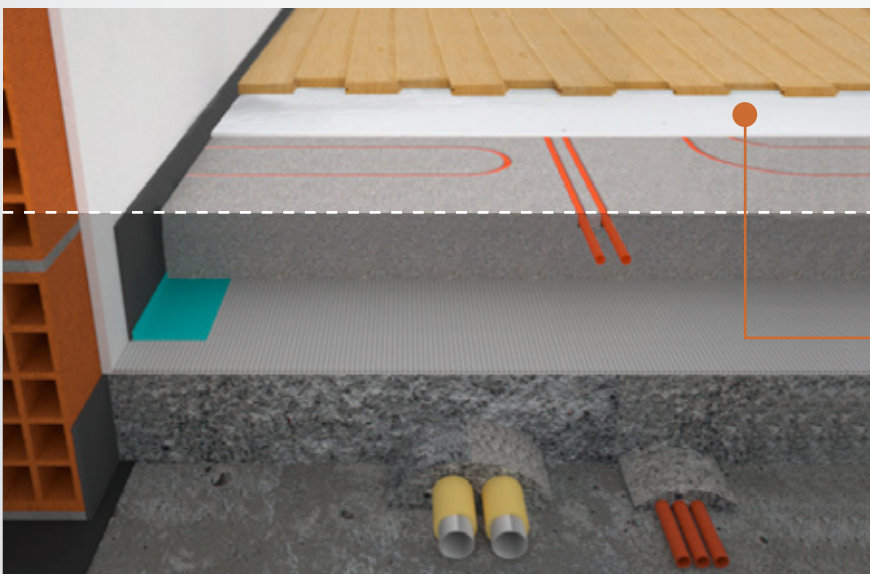
POSA FLOTTANTE DI PAVIMENTI IN LEGNO, LAMINATI O LVT
